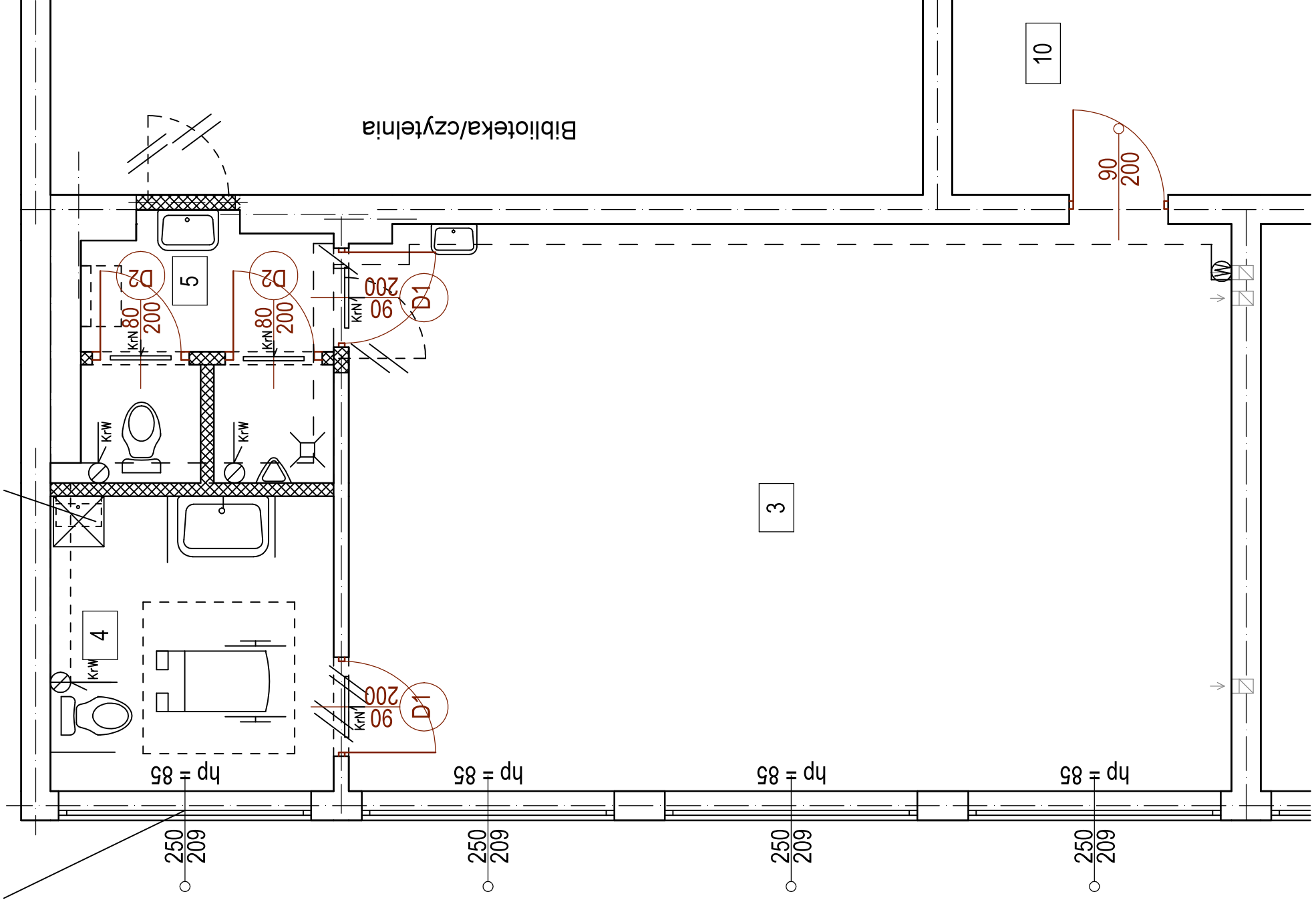
Plan instalacji wentylacji WC 1:50
