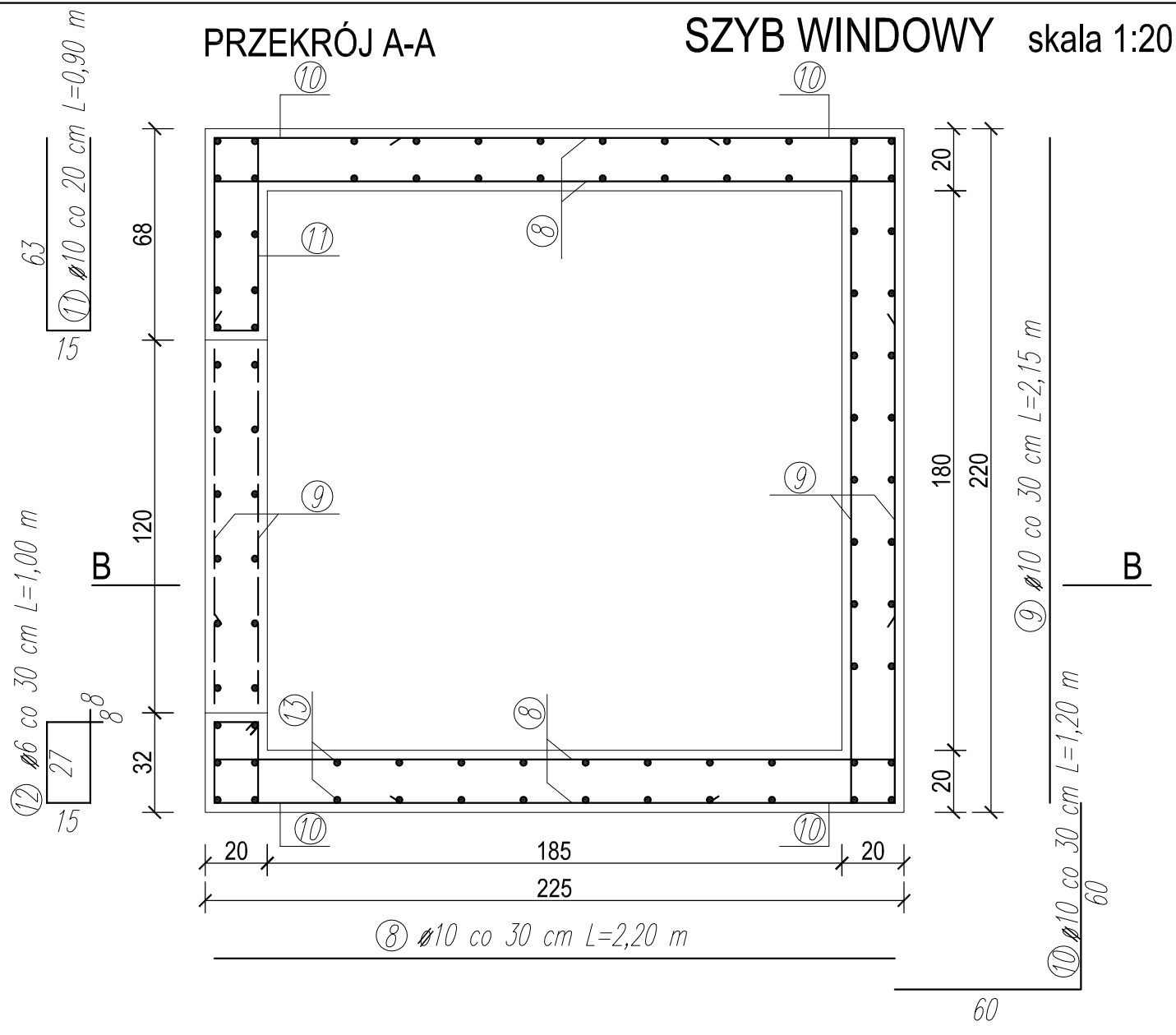
WYKAZ STALI ZBROJENIOWEJ / 18G2
