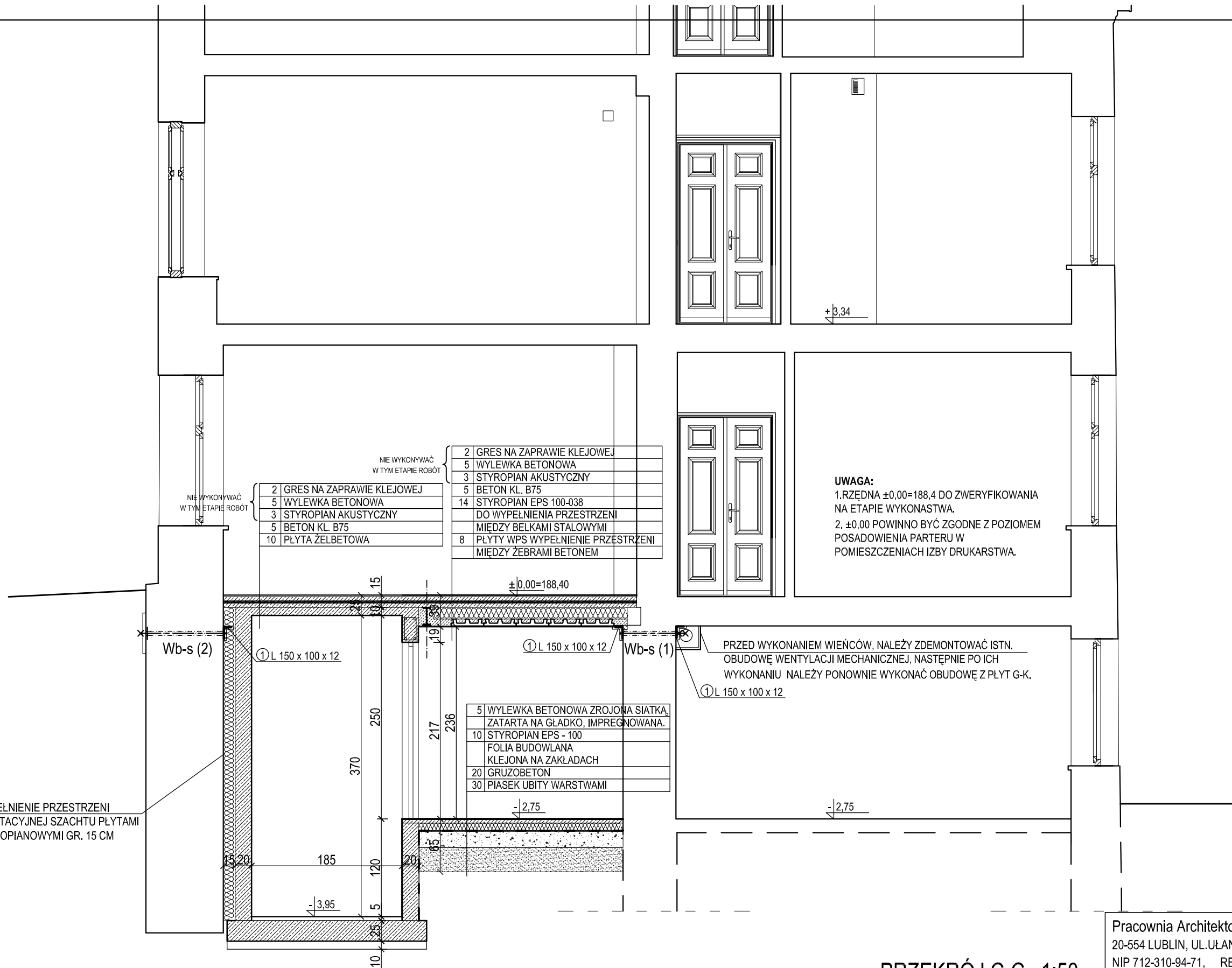
PRZEKRÓJ C-C 1:50
