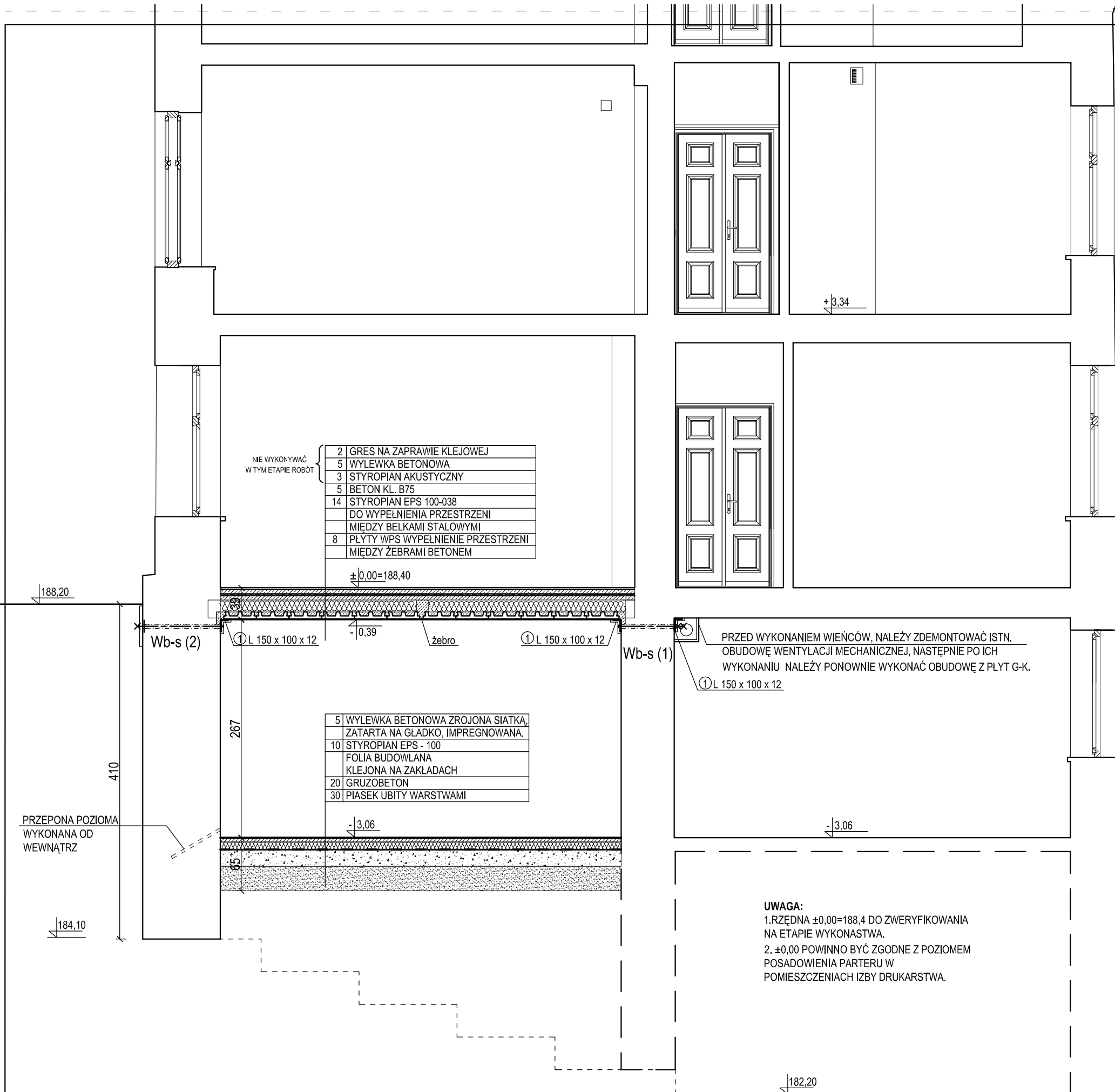
PRZEKRÓJ A-A 1:50
