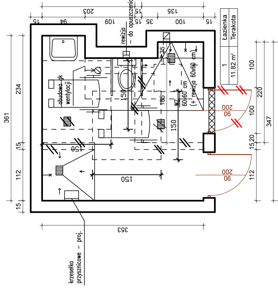
Projekt – łazienka II piętro 1:50
