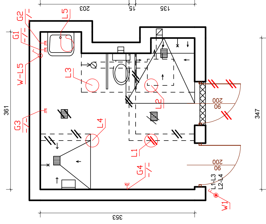
Projekt – łazienka II piętro 1:50 schemat instalacji elektrycznych
