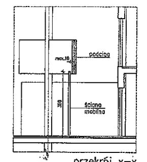
przekrój x-x
